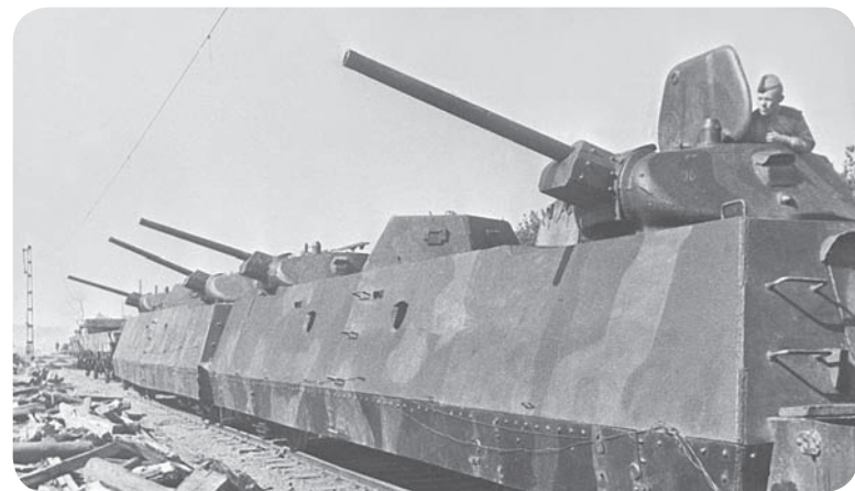
Бронеплощадки построенные по проекту бронеплощадок Особого бронепоезда № 1 «За Сталина» на боевой позиции.
