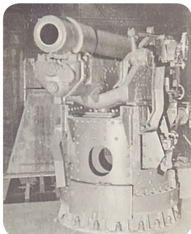
152 мм гаубица системы «Виккерс» образца 1916 г. бронепоезда «Коломенский рабочий». Оригинал фотографии хранится в музее АО «Коломенский завод».
