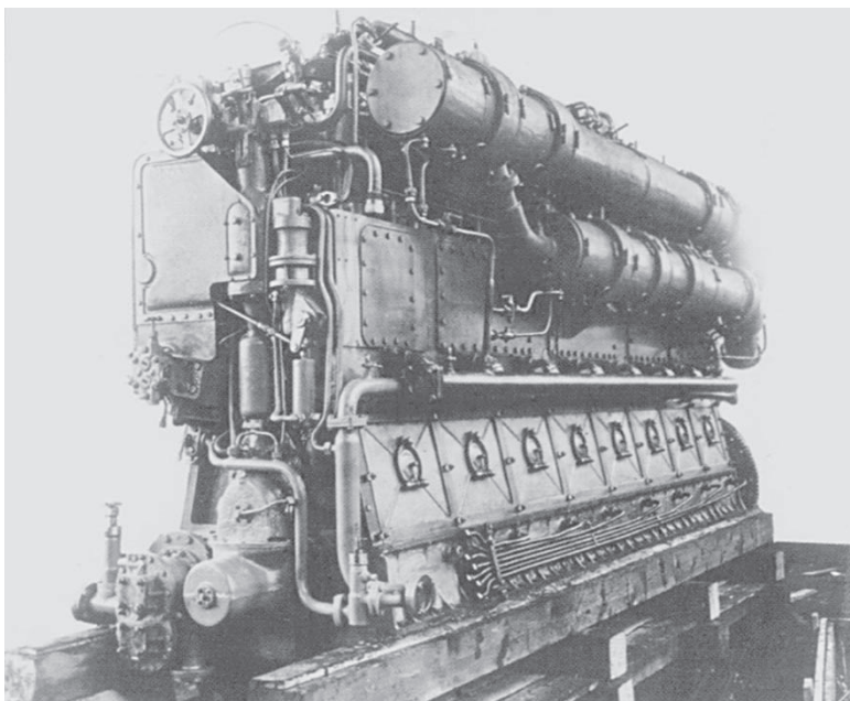
Дизель 1Д. Этими двигателями оснащались подводные лодки типа «С» («Сталинец») и «Л» («Ленинец»). Два подобных дизеля стояли на подлодке «С-13», которой командовал А. И. Маринеско.
