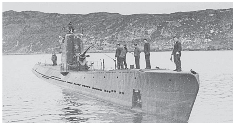
Подводная лодка «С-56» возвращается из третьего боевого похода. 21 июля 1943 г.
