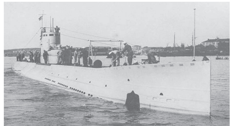
Подводная лодка Л-4 «Гарибальдиец» типа «Ленинец» с дизелем 42БМ6.
