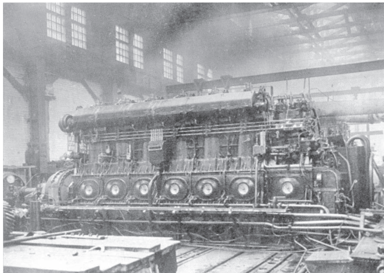
Дизель 42БМ6 для подводных лодок типа «Декабрист» и «Ленинец». В предвоенный период дизели марки 42БМ6 были установлены на 4 ПЛ типа «Декабрист» и 19 ПЛ типа «Ленинец». На каждой субмарине было по два двигателя. Фотография сделана на Коломенском заводе.
