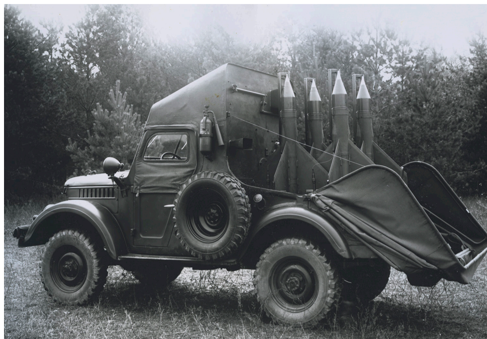
Боевая машина 2П26 с противотанковым комплексом «Шмель»
